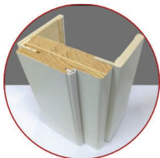
Telaio Listellare spessore da 85 a 120 mm, coprifili 70/90 in multistrato
